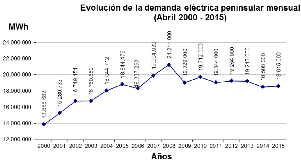
Gráfica 3. Evolución demanda eléctrica del Sistema Peninsular. Cifras actualizadas por WWF a 04/05/2015.
