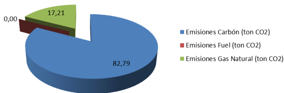
Gráfica 5. Origen de emisiones de CO2 de centrales térmicas. Fuente: REE y elaboración propia.
