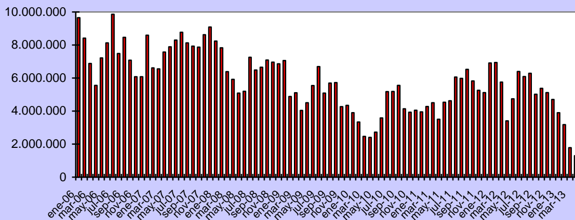
Evolución emisiones mensuales CO 2 generación eléctrica peninsular ( 2006-2013, no incluye cogeneración)
