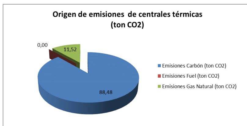
Gráfica 5. Origen de emisiones de CO 2 de centrales térmicas. Fuente: REE y elaboración propia.
