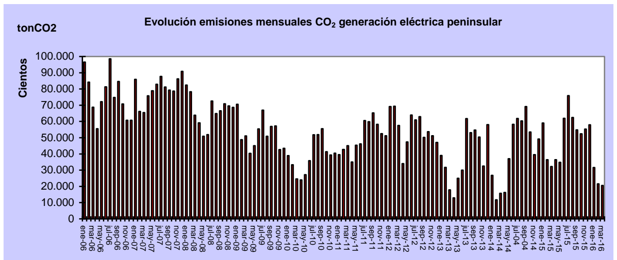
Gráfica 3. Fuente: REE y elaboración propia.
