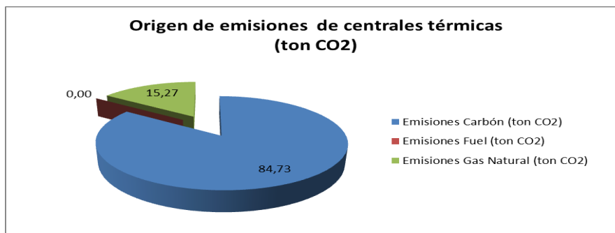
Gráfica 5. Origen de emisiones de CO 2 de centrales térmicas. Fuente: REE y elaboración propia.
