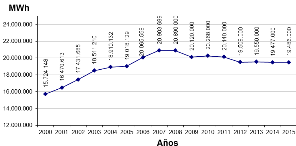
Gráfica 3. Evolución demanda eléctrica del Sistema Peninsular. Cifras actualizadas por WWF a 02/11/2015.
