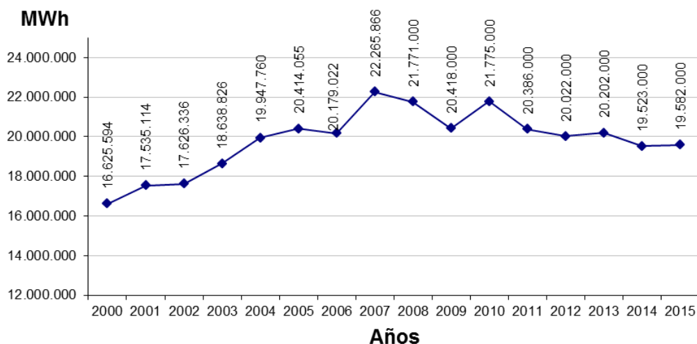
Gráfica 3. Evolución demanda eléctrica del Sistema Peninsular. Cifras actualizadas por WWF a 05/10/2015.
